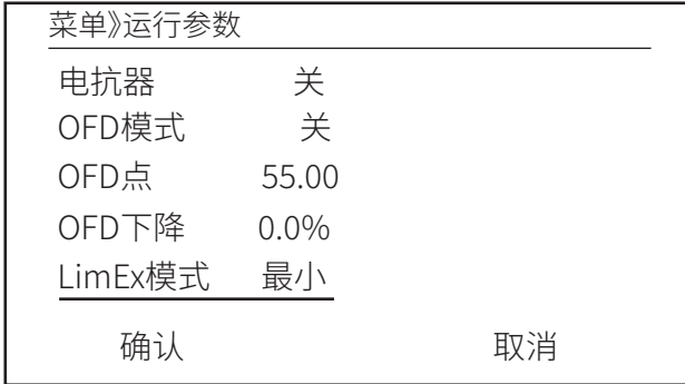
图8.15.1 功能
