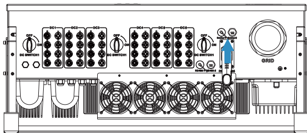
图5.14 数据采集器的安装
