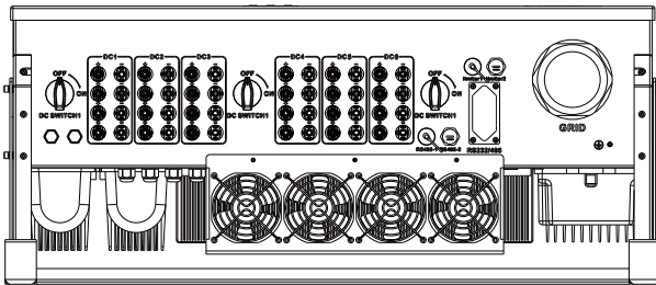
图1.2 底视图
