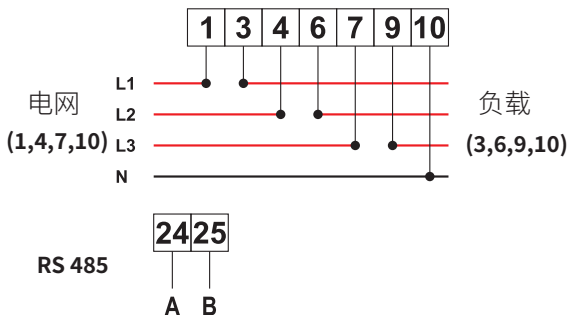
图7.5 正泰电表
